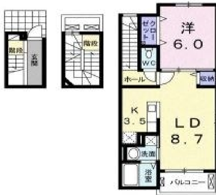
【間取り図】
